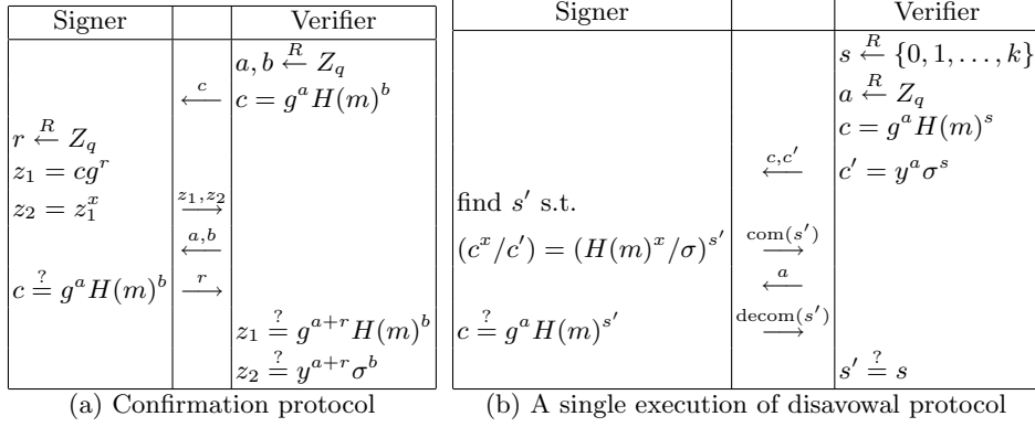
Fig. 1. ZKIP protocols
