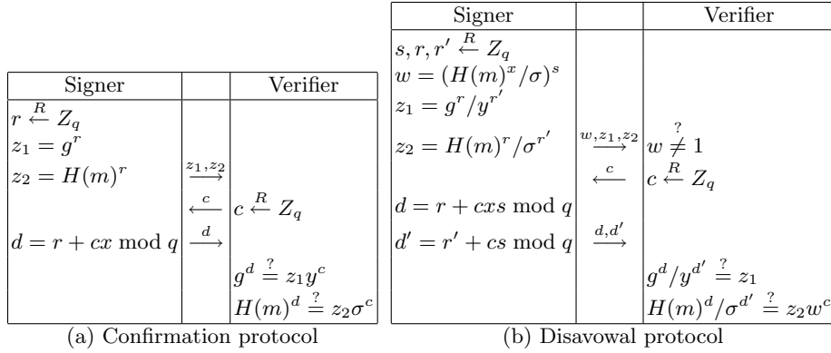
Fig. 2. HVZK protocols
